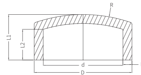
(SOCKET WELD)
