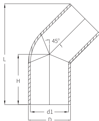
(BUTT WELD)
