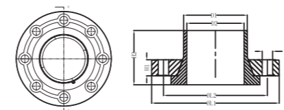
(BUTT WELD)
