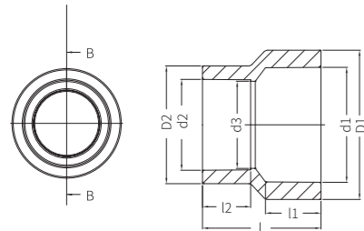
(SOCKET WELD)
