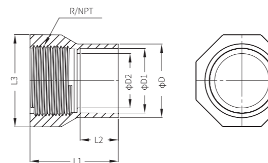
(BUTT WELD)
