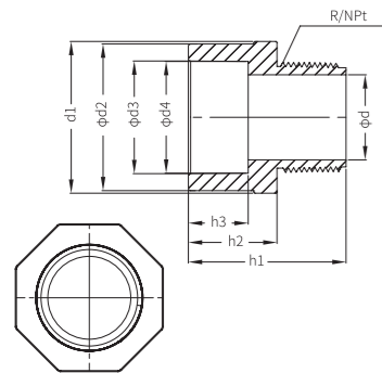
(SOCKET WELD)
