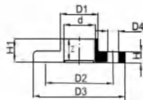
(SOCKET WELD)
