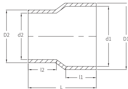
(BUTT WELD)
