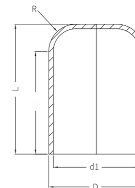
(BUTT WELD)
