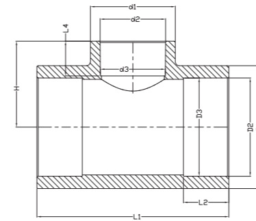
(SOCKET WELD)
