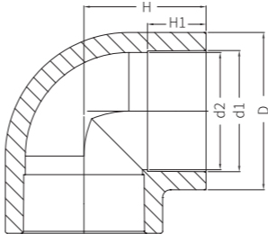
(SOCKET WELD)
