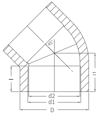
(SOCKET WELD)
