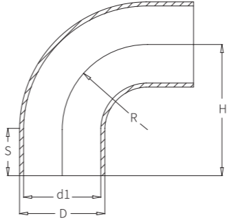
(BUTT WELD)
